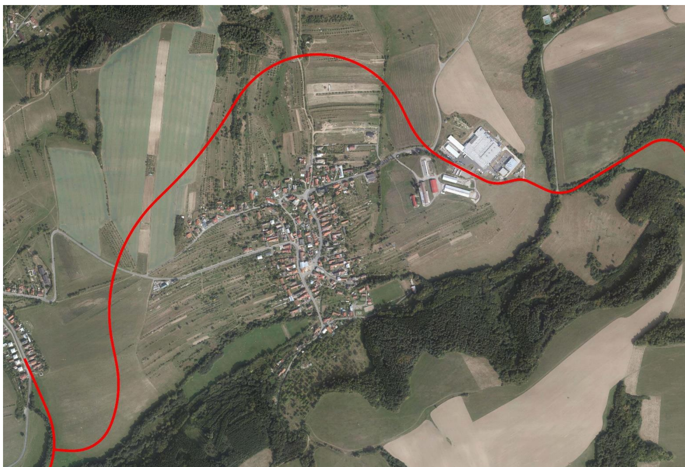
Navržená trasa vyhledávací studie přeložky komunikace Vysoké Pole - Drnovice
